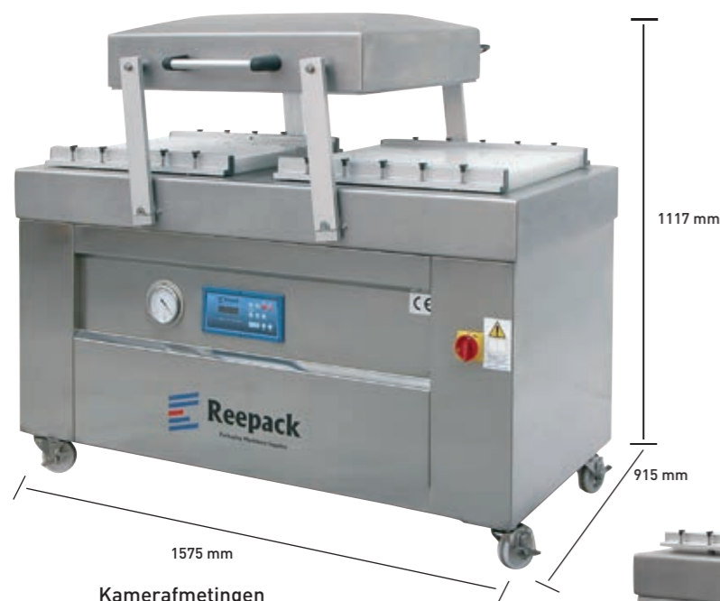
Kamerafmetingen Dimensions de la chambre 808 x 200 x 730 mm (wxhxd)
